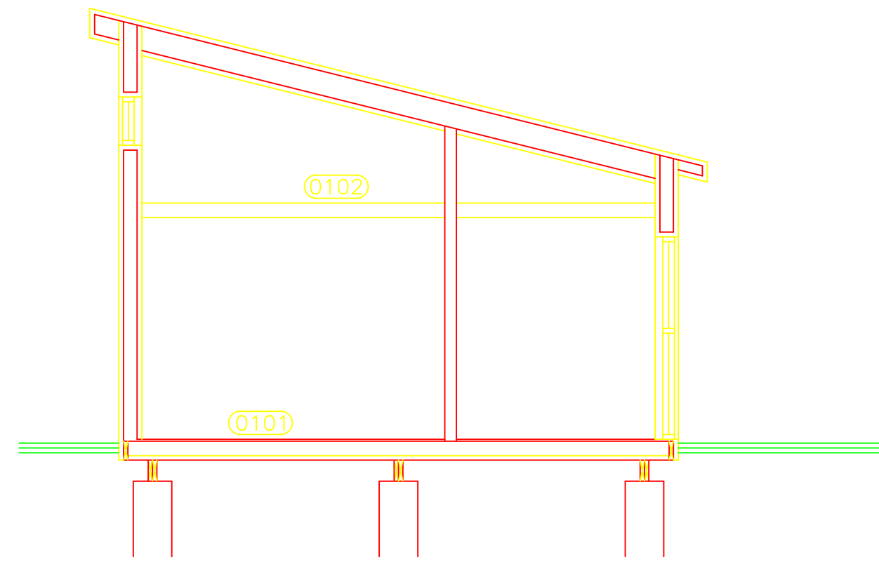
Sneiðing A 1:100
