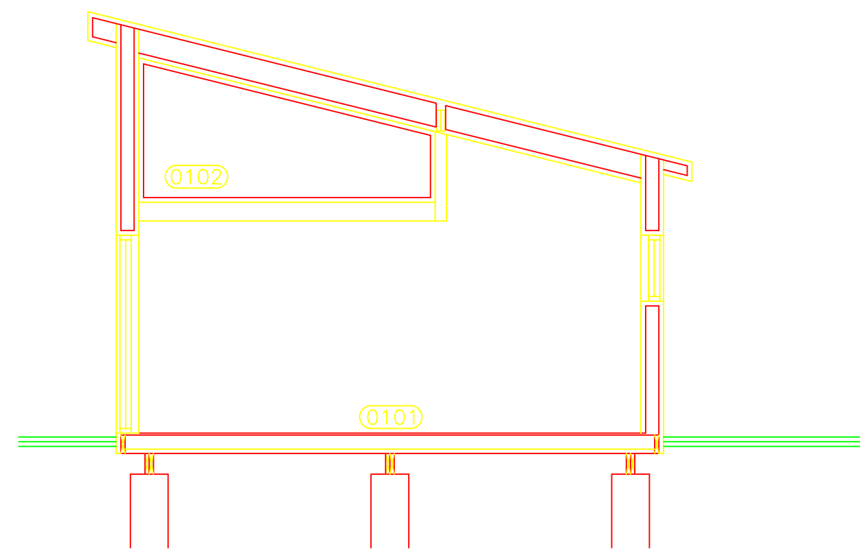
Sneiðing C 1:100
