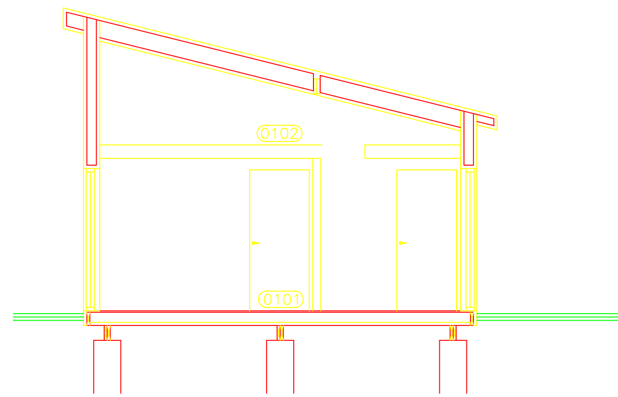
Sneiðing B 1:100
