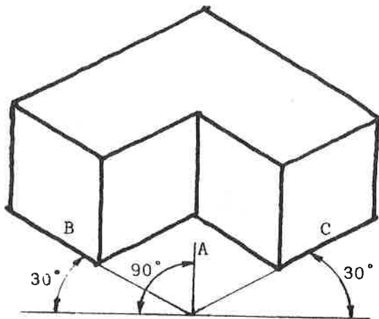
A:B:C = 1:1:1 Samkvarðamyndun (ísómetrí)
